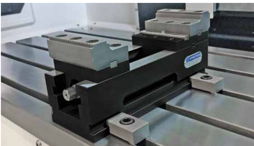
Mechanische Kompaktspanner MSU 280-100 mit Grip-Wendebacken Mechanical compact vises MSU with reversible grip jaws
